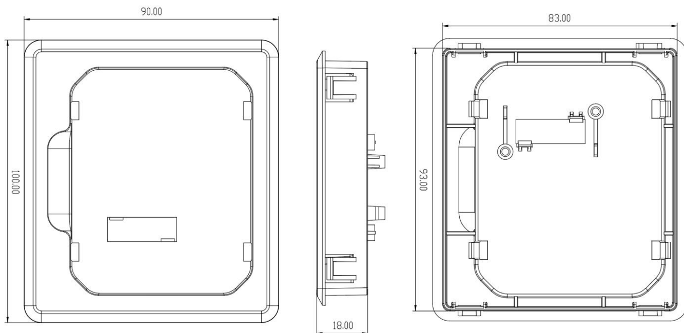
通用款托盘外形尺寸图
