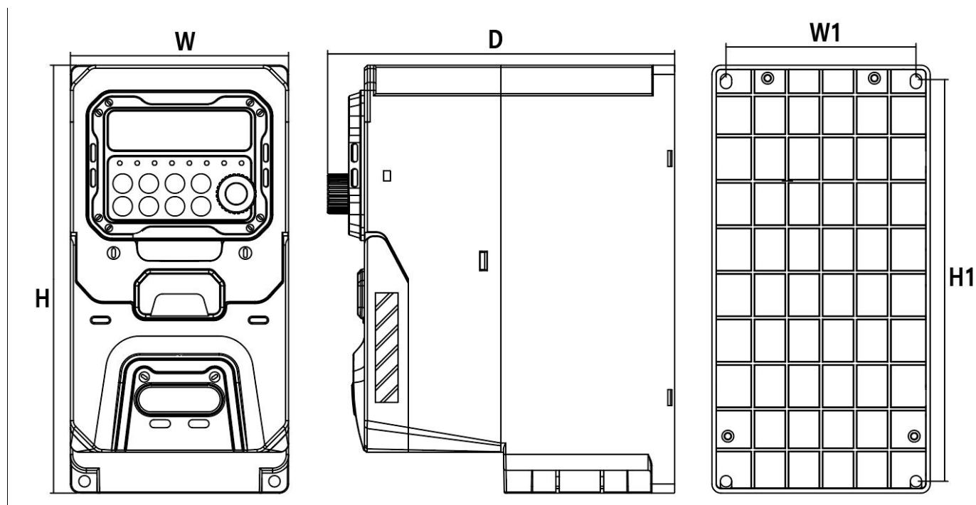
通用款外形尺寸图
